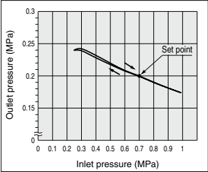
AW30-A
