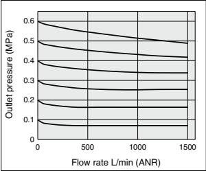
AW30-A Rc3/8
