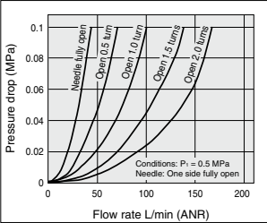
AL40-A Rc1/2
