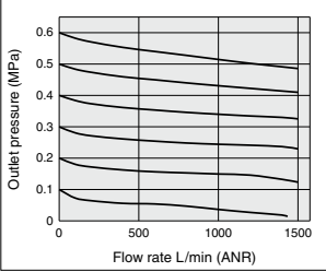
AC30-A Rc3/8
