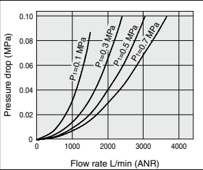
AF50-A Rc1
