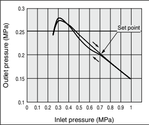
AC30-A
