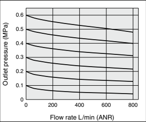
AC40-A Rc1/2
