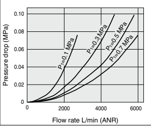
AF40-06-A Rc3/4
