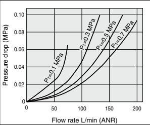
AF40-A Rc1/2
