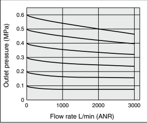
AW40-A Rc1/2
