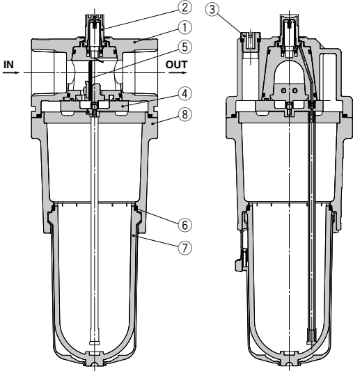
AL50-A/AL60-A
