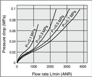
AL40-06-A Rc3/4
