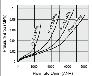
AL60-A Rc1
