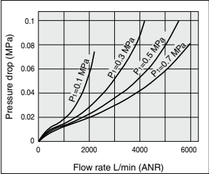
AL50-A Rc1
