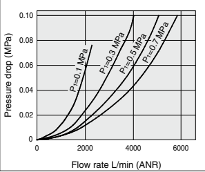
AF60-A Rc1
