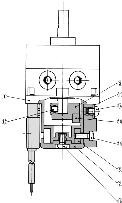
CDRB2BW20, 30-□ S D
