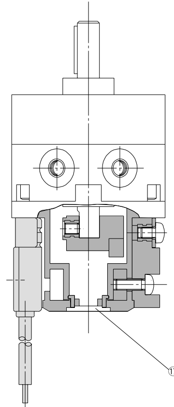
CDRB2BW40-□ S D
