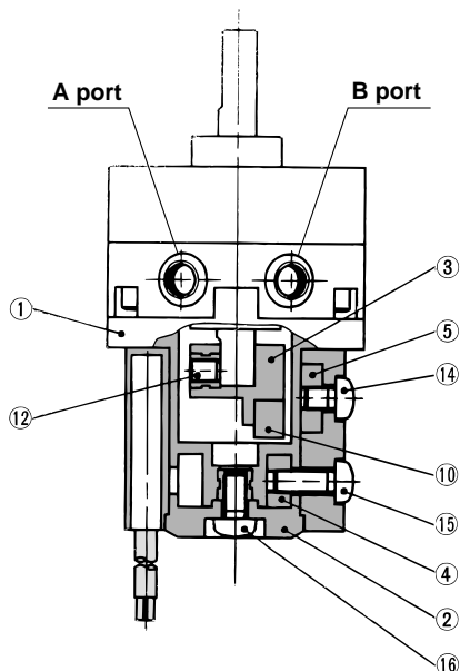
CDRB2BW10, 15-□ S D
