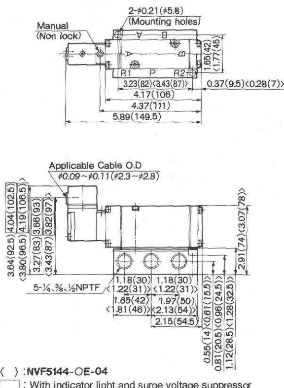
DIN Connector/NVF5144-OD
