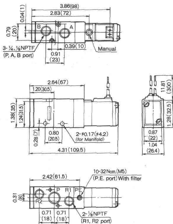
Grommet/NVF3130-OG
