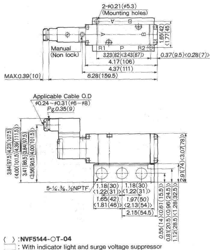
Conduit Terminal/NVF5144-OT
