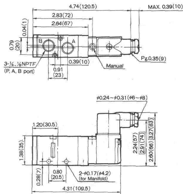
DIN Connector/ NVF3130-OD
