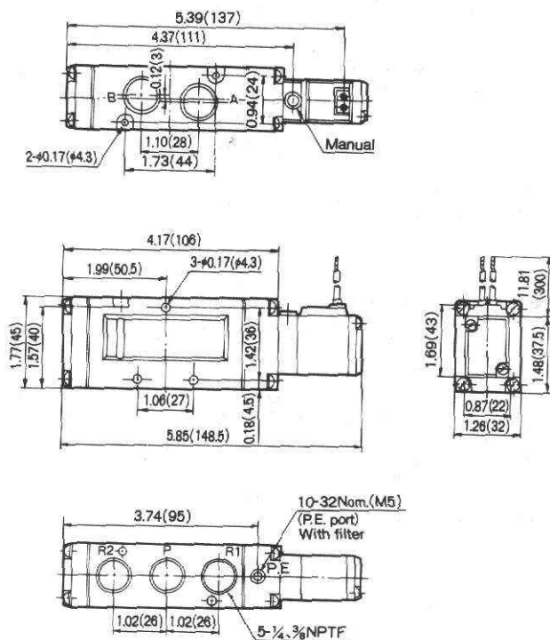
Grommet/NVF5120-OG
