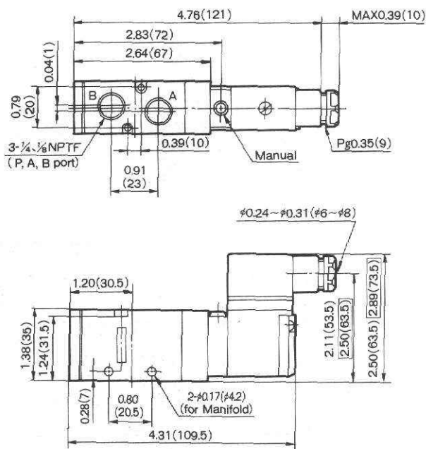
Conduit Terminal/ NVF3130-OT
