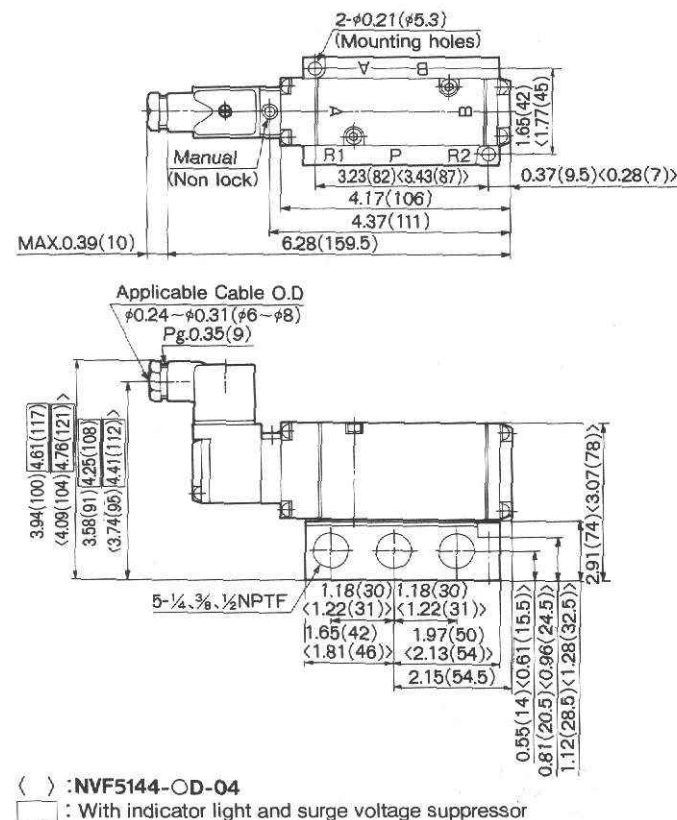
DIN Connector/NVF5144-OD
