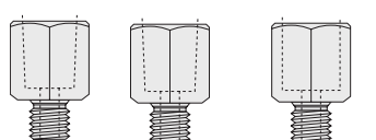
10-32x1/16-F 10-32x1/16BSPT-F 10-32x1/16BSPP-F
