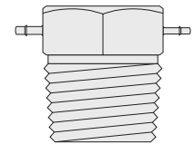
3/8RT.040-.031
