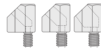
8-32x10-32-FL-45° 10-32x4-28-FL-45° 10-32x1/8-FL-45°
