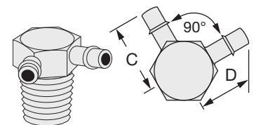
1/8 VT6-90°
