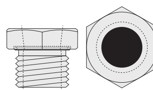
RB9/16-18-SAE x 1/4
