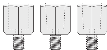
10-32x1/8BSPP-F 10-32x1/8-F 10-32x1/8BSPT-F
