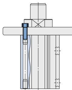
Rod end tapped
