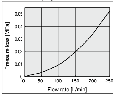
PF3W721(-L)
