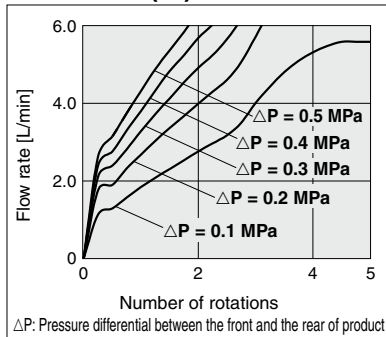
PF3W704S(-L)/504S
