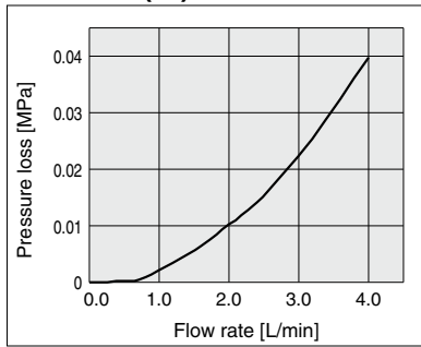
PF3W711(-L)/511
