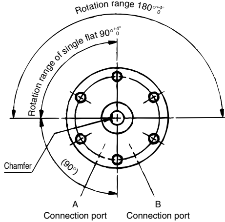
Single vane: 90°, 180°
