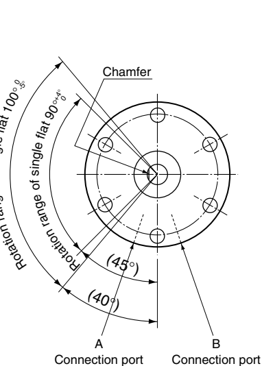
Double vane: 90°, 100°
