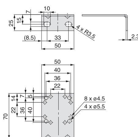
L-bracket
