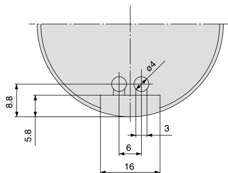
MSH3-50DA
